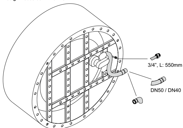
Připojovací rozměry pro odtokovou a přepadovou soustavu
