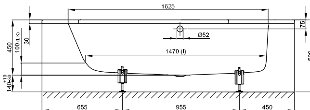
N° 2: obj. č. 6841, strana nohou vlevo, přepad vpředu
