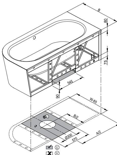
Připojovací rozměry pro odtokovou a přeпадovou soustavu
