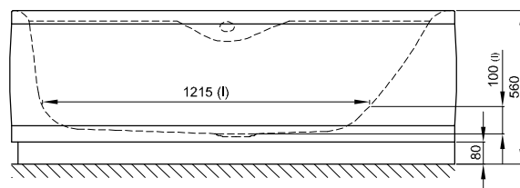
N° 2: Roh pravý, obj. č. 6053 CELV
