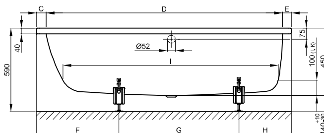
N° 2: strana nohou vpravo, přepad vpředu
