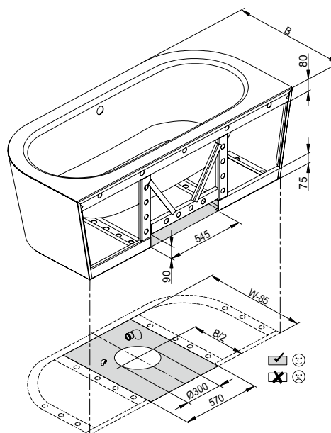
Připojovací rozměry pro odtokovou a přečpádovou soustavu
