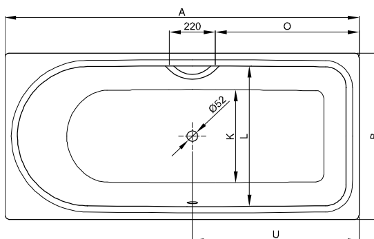
N° 2: strana nohou vpravo, přepad vpředu
