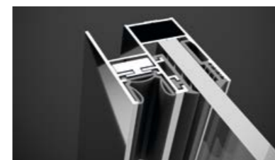
Stěnový profil poskytuje nastavitelnost až 20 mm pro vyrovnání nerovností. Zároveň přidržuje dveře v otevřené pozici.
