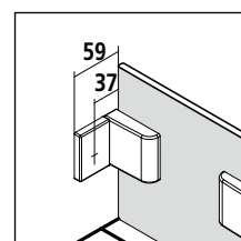
Stěnový pant venku
